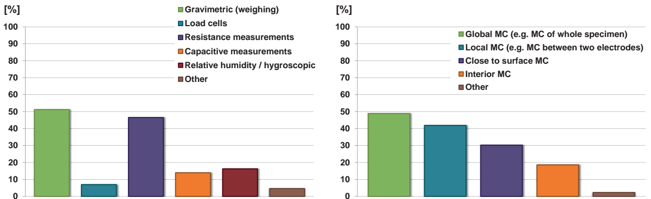
Abbildung 3: Ergebnisse der PerformWOOD Web-Befragung. Links: Methoden zur Holzfeuchtebestimmung im Freiland. Rechts: Arten der Holzfeuchte, die bestimmt werden.
