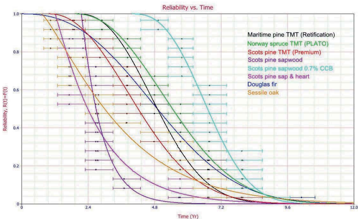
Abbildung 4: Verlässlichkeit und Standardabweichung der Abbaubewertung für unterschiedliche Holzarten und Behandlungen nach Prüfung im Erdkontakt (EN 252, 1989) am Standort Hamburg (aus: Van den Bulcke et al. 2013).
