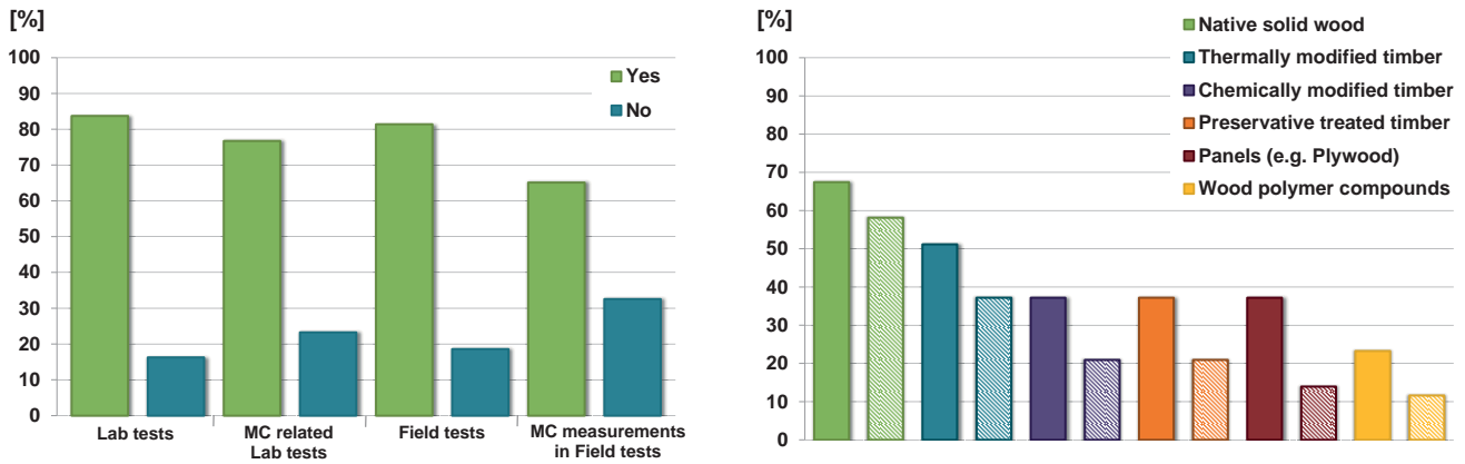
Abbildung 2: Ergebnisse der PerformWOOD Web-Befragung. Links: Durchgeführte Prüfmethode. Rechts: Materialien die hinsichtlich ihrer Feuchte-Performance geprüft werden (Labor- und Freilandprüfungen), vollfarbig: Laborprüfungen, gestrichelt: Freilandprüfungen.
