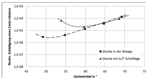
Abb. 6: Auswirkung der Ausrichtung einer Glocke am Joch auf das Risiko von Schäden
