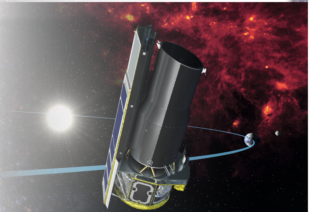
Spitzer-Weltraum-Teleskop / NASA
