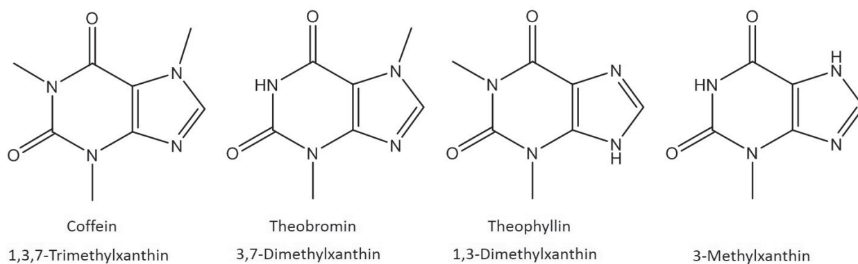
Abbildung 2-3: Strukturformel der in dieser Arbeit untersuchten Xanthinderivate
