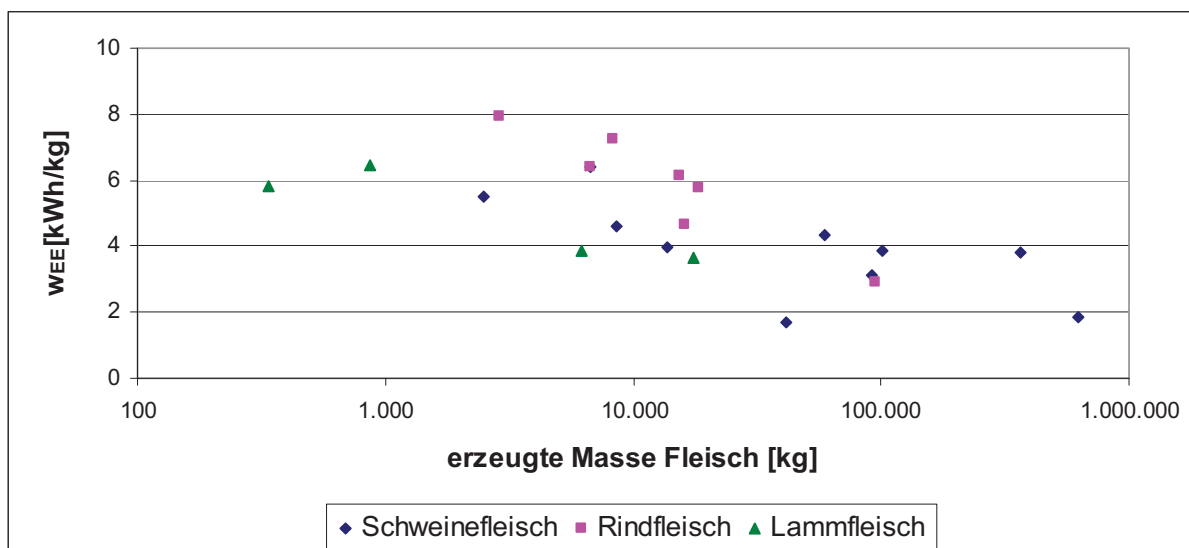
Abb. 5-19: Spezifische EEU der Fleischbereitstellung über der Betriebsgröße
